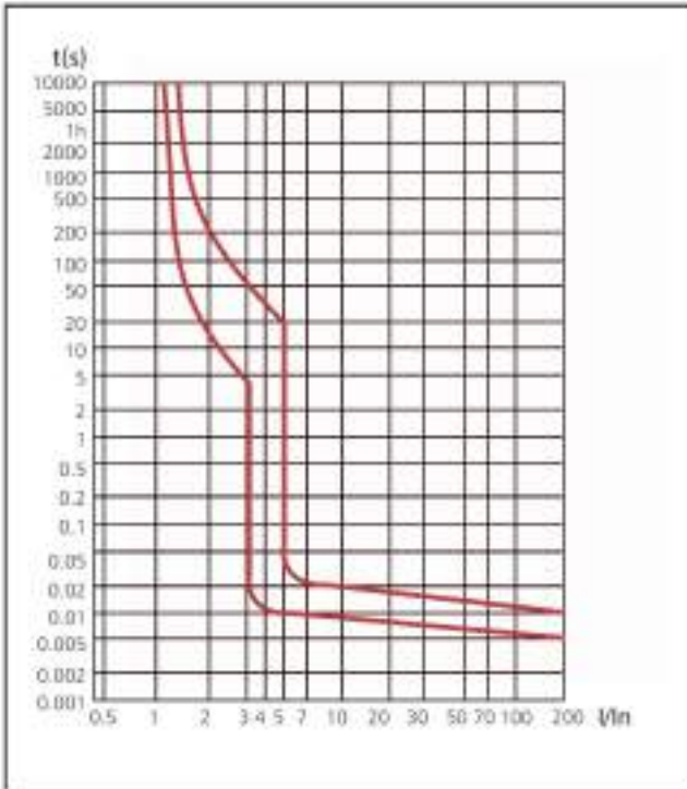
Kennlinie B
