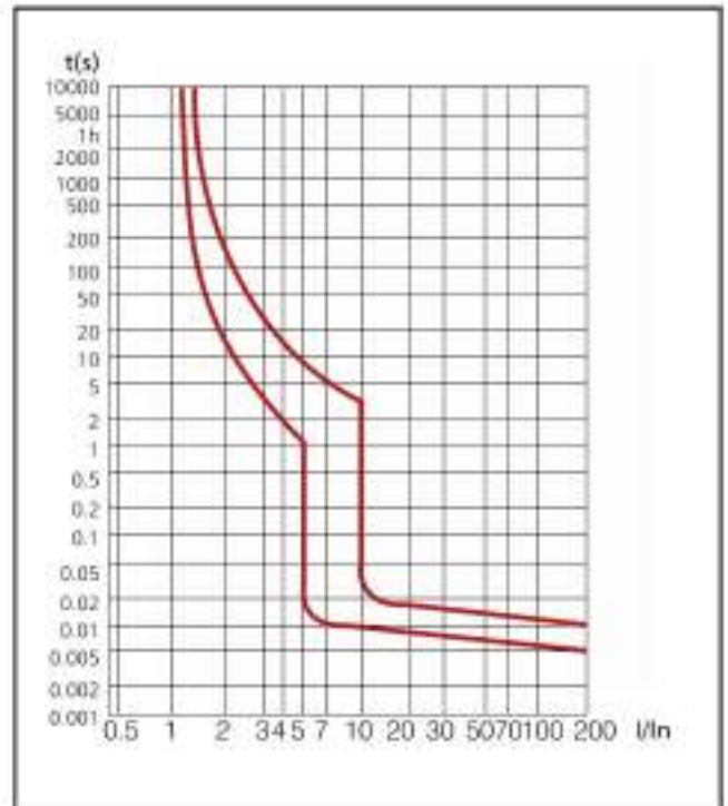
Kennlinie C
